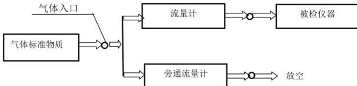
图 1 仪器气路连接示意图
